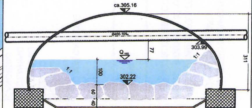
ATTRAVERSAMENTO COLLETTORE CONSORTILE ESISTENTE NEL RIALE TERSAGGIO PROGETTATO
